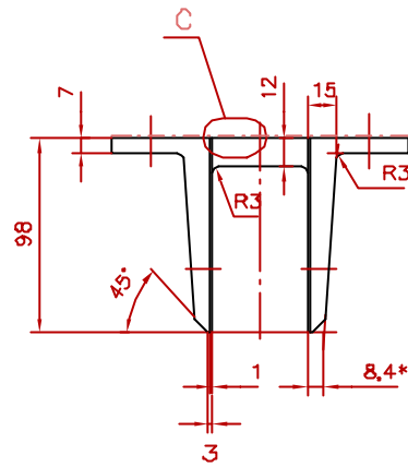
A-A(1:1)
