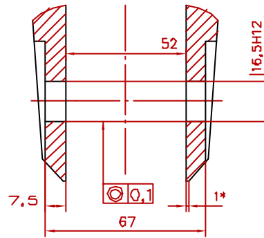
A-A(1:1)
